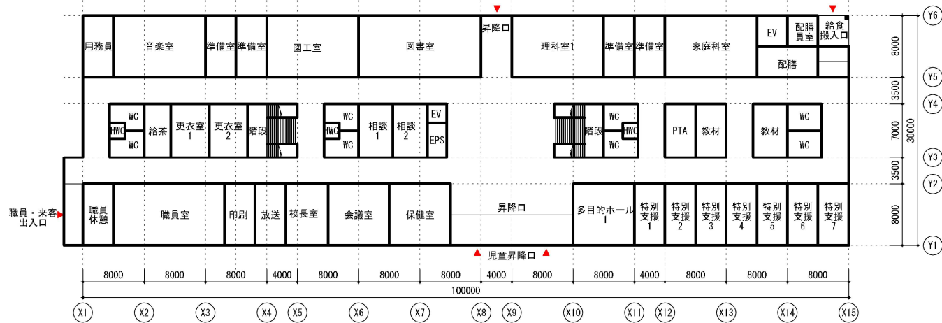
1階平面図 A3:1/500
