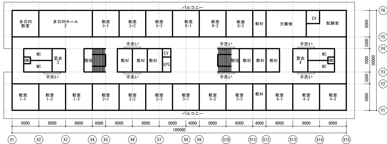
2階平面図 A3:1/500
