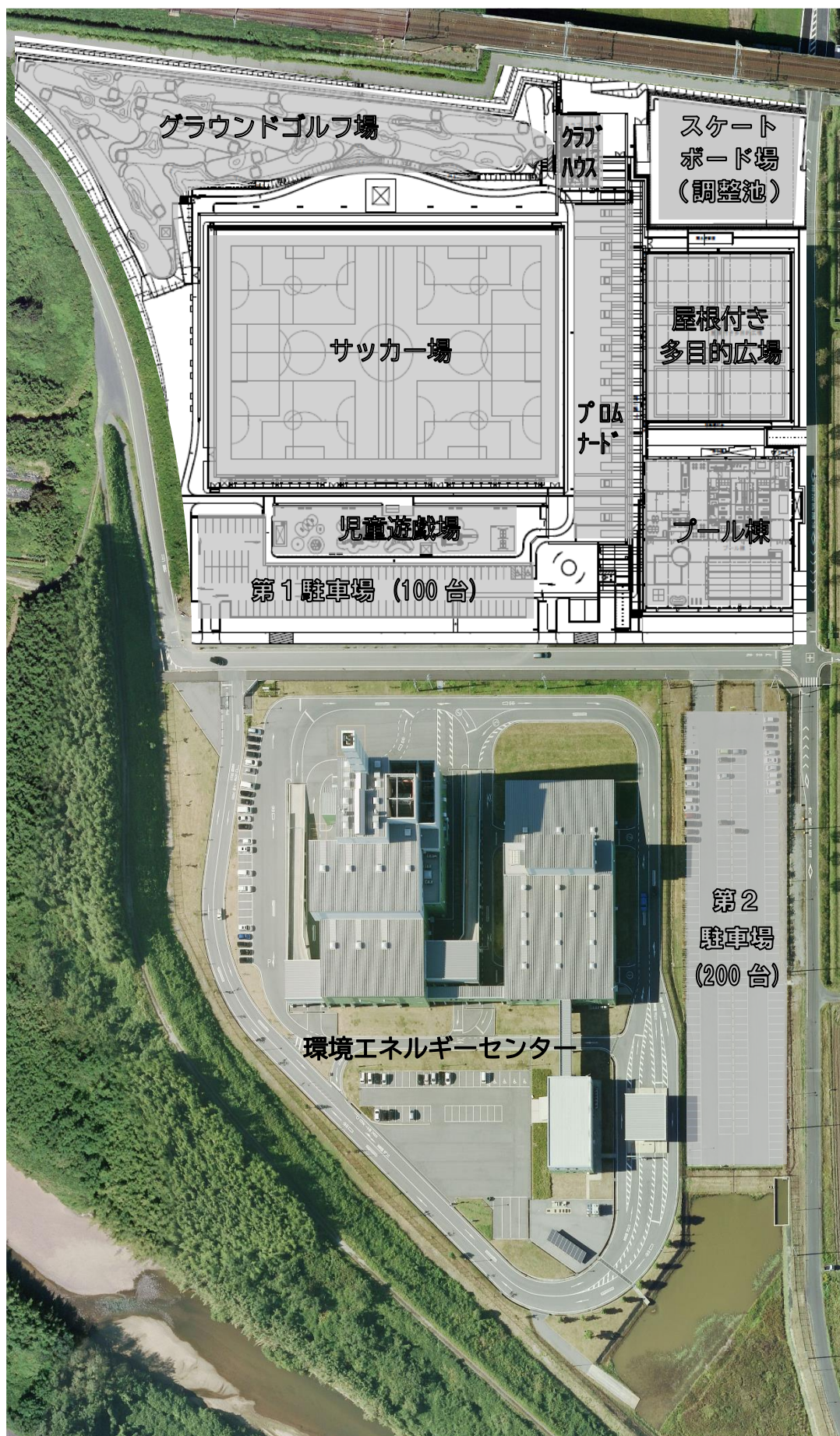
【配置図】
