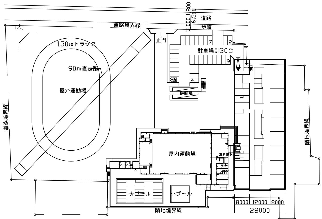
現地整備案 岡山小校舎規模
