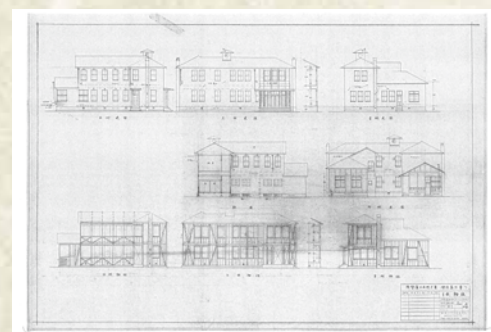
旧八幡警察署（市立資料館）改築立面図
